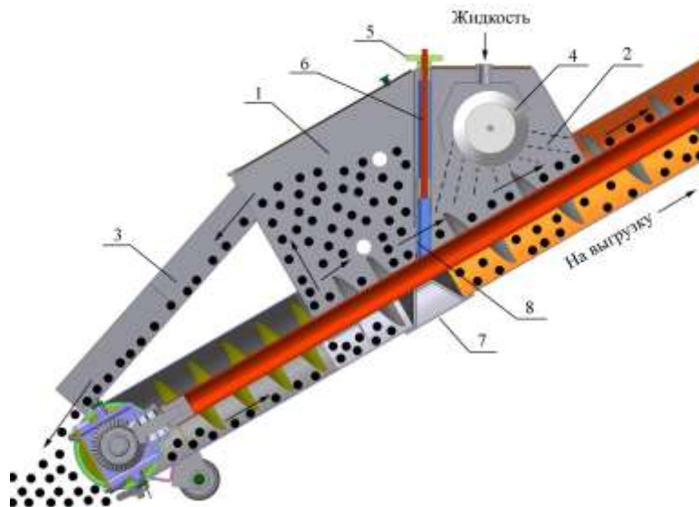
Технологическая схема ПК-10:
